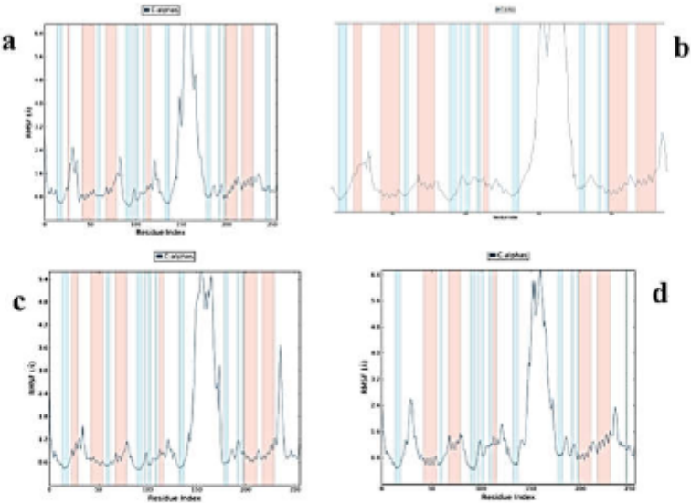
Fig. 8. RMSF of a: Apo-state of caspase -8; b: carnosol-caspase-8; c: luteolin-caspase-8; d: melphalan-caspase-8
