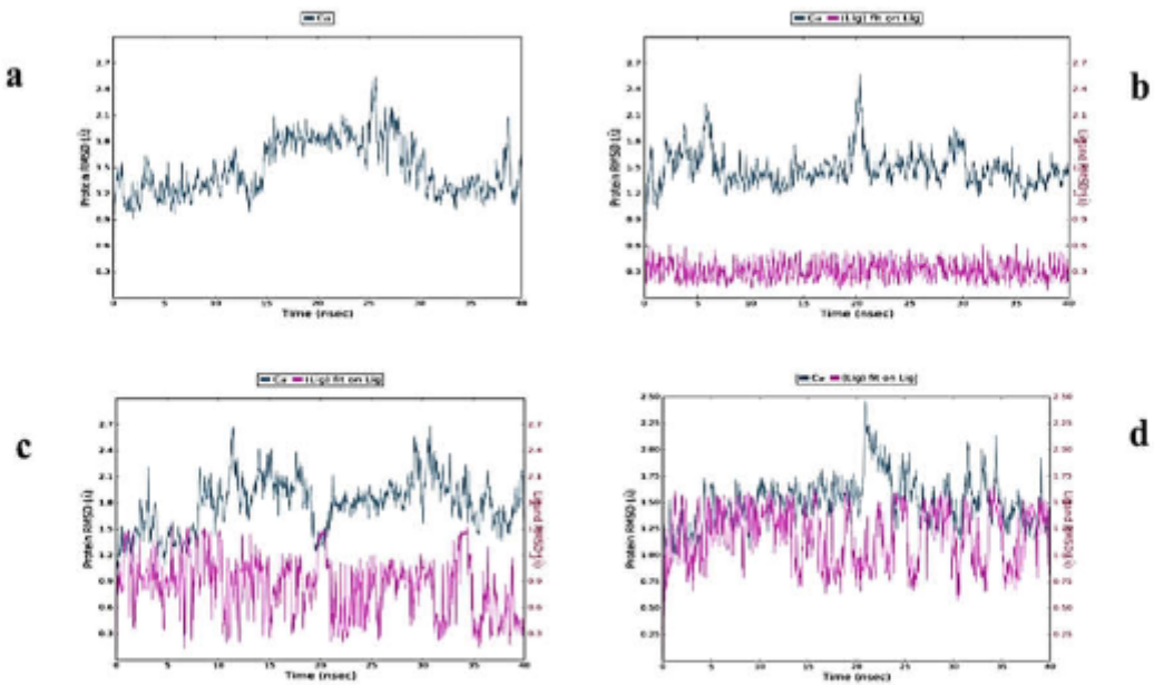
Fig. 5. RMSD of a: Apo-state of caspase -3; b: carnosol-caspase-3; c: luteolin-caspase-3; d: melphalan-caspase -3
