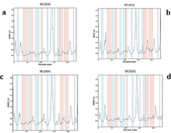
Fig. 7. RMSF of a: Apo-state of caspase -3; b: carnosol-caspase-3; c: luteolin-caspase-3; d: melphalan-caspase -3
